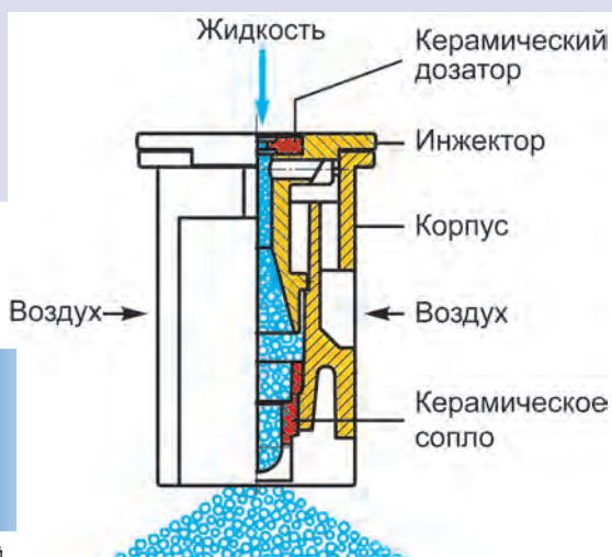
съёмный инжектор
