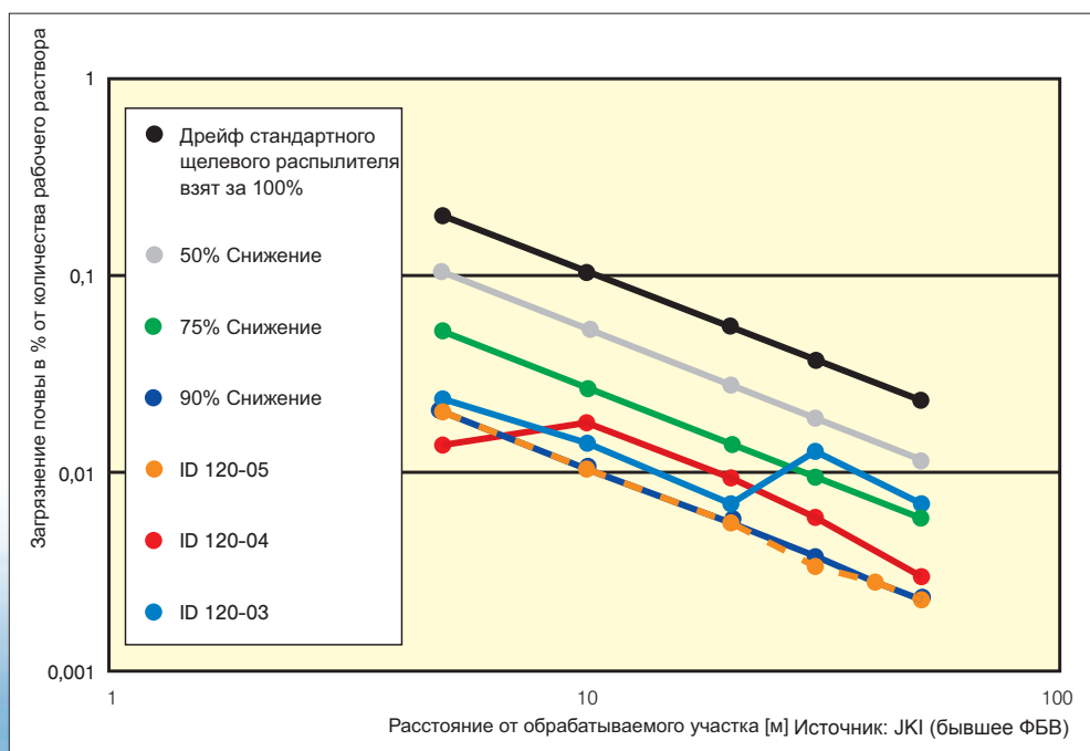
Уменьшение сноса при применении инжекторных распылителей ID по сравнению с выведенным пограничным значением (полеводство), полученным на обычных щелевых распылителях
